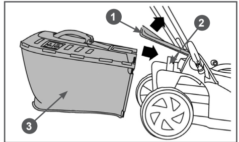
Рис. 7 Установка травосборника
