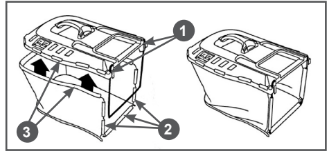
Рис. 6 Сборка травосборника
